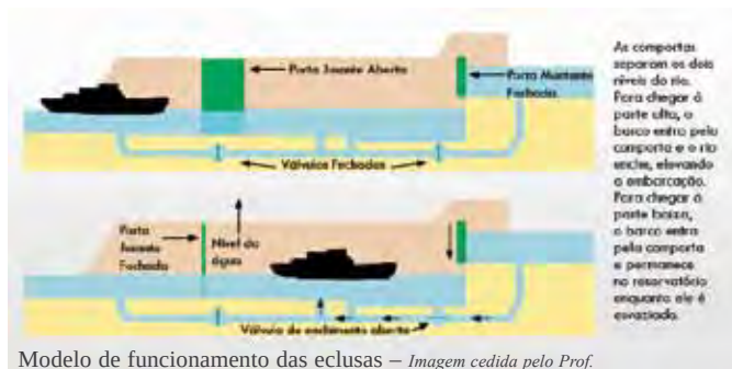
Modelo de funcionamento das eclusas – Imagem cedida pelo Prof. Hito Braga de Moraes
